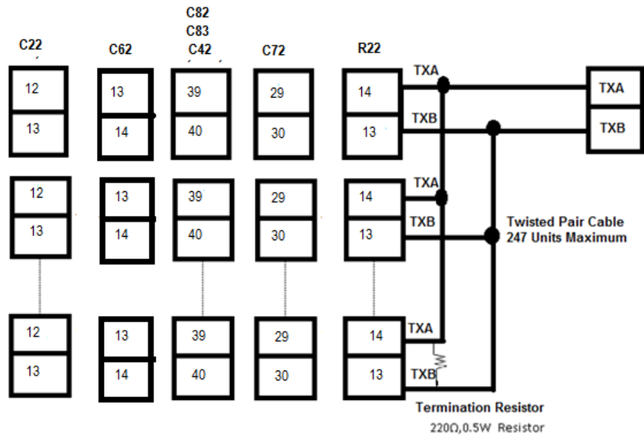
2-42 RS-485 Wiring
